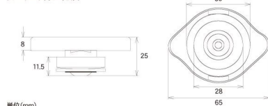
ラジエターキャップ寸法図
